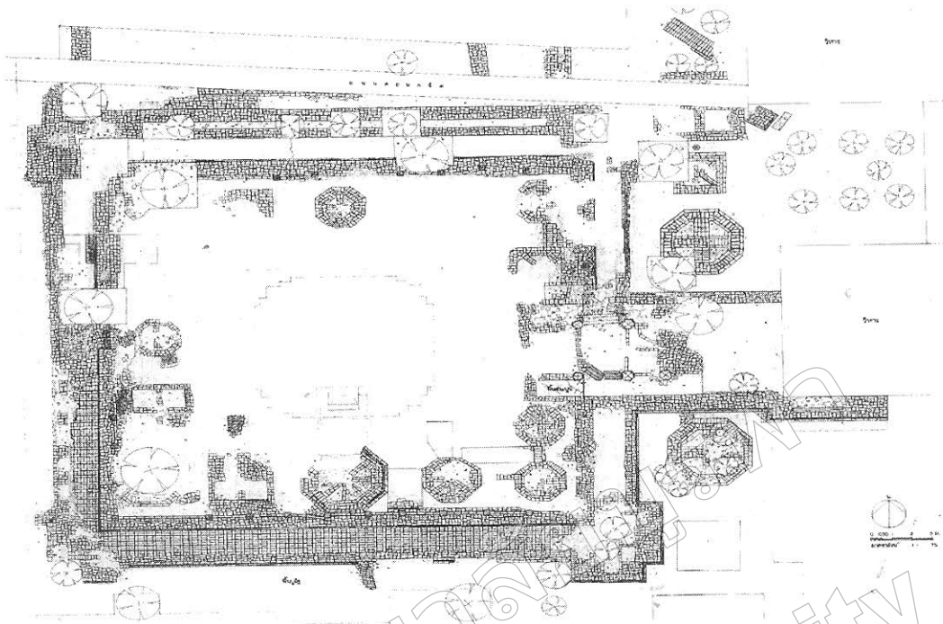
4. แผนผัง จัดทำจากหลักฐานการขุดแต่ง ระเบียงคด เจดีย์ประธาน เจดีย์บริวาร และวิหารซึ่งท้ายยื่นผ่านยานกลางของระเบียงคดด้าน ตะวันออก (ภาพจาก "รายงานการขุดแต่งทางโบราณคดี โบราณสถานวัดสองพี่น้อง, 2554).
