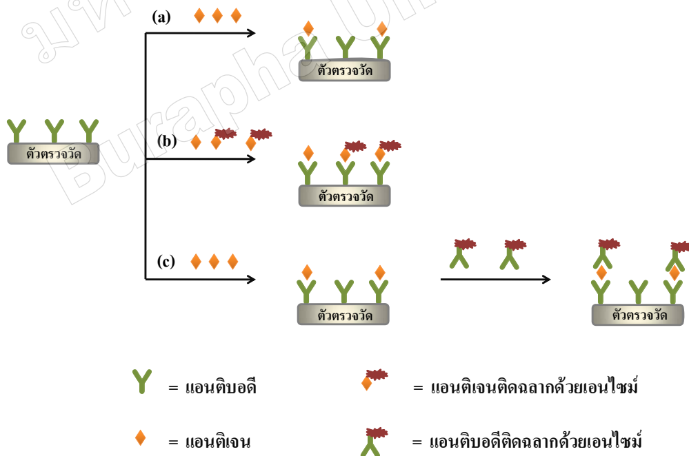
ภาพที่ 3 ประเภทของอิมมูโนเซนเซอร์ โดยตรงแอนติบอดีไว้บนตัวตรวจวัด เพื่อวิเคราะห์หาปริมาณแอนติเจน (a) แบบตรง สามารถวิเคราะห์หาแอนติเจนได้โดยตรง (b) แบบแข่งขัน โดยใช้แอนติเจนติดฉลากด้วยแอนไซม์ และ (c) แบบแซนดวิช อาศัยการตรวจวัดจากแอนติบอดีที่ติดฉลากด้วยแอนไซม์ (Ricci et al. , 2007)
