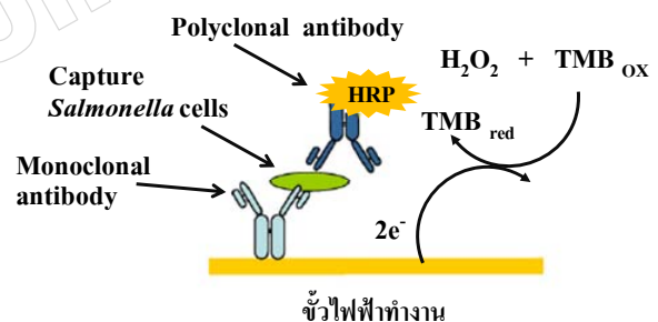
ภาพที่ 4 อิมมูโนเซนเซอร์แบบแซนด์วิช เพื่อวิเคราะห์หาปริมาณ Salmonella โดยติดฉลากแอนติบอดีด้วยเอนไซม์ HRP และใช้ H_2O_2 เป็นสารช่วยส่งผ่านอิเล็กตรอน ผลจากปฏิกิริยาของเอนไซม์จะได้กระแสไฟฟ้าเกิดขึ้น และสามารถตรวจวัดด้วยเทคนิคแอมเพอร์โรเมตริก (ที่มา: Salam et al. , 2009)
