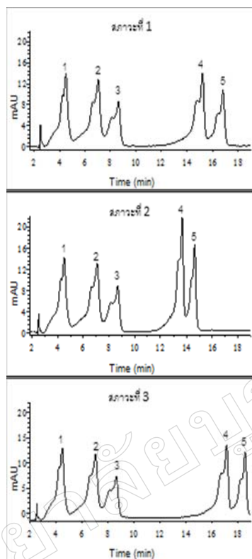
ภาพที่ 2 โครมาโทแกรมการแยกสารซัลโฟนาไมด์ 5 ชนิด ภายใต้สภาวะการแยกที่ 1, 2 และ 3 (สภาวะตามตารางที่ 1) โดยพีคที่ 1: ซัลฟาเมธอกซี, 2: ซัลฟาคลอโรไพริดาซีน, 3: ซัลฟีโซซาโซล, 4: ซัลฟาไดเมธอกซี และ 5: ซัลฟาควินอกซาไลน์
