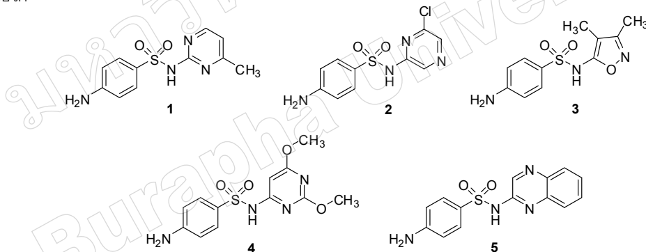
ภาพที่ 1 โครงสร้างของซัลฟาเมอราซีน (1), ซัลฟาคลอโรไพริดาซีน (2), ซัลฟิโซซาโซล (3), ซัลฟาไดเมธอกซีน (4) และซัลฟาควินอกซาไลน์
