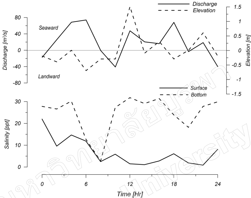
ภาพที่ 4 การเปลี่ยนแปลงตามวัฏจักรน้ำขึ้นน้ำลงของระดับน้ำและฟลักซ์ของน้ำ (บน) และความเค็มบริเวณใกล้ผิวน้ำและพื้นที่ท้องน้ำ (ล่าง) บริเวณปากแม่น้ำระยองในช่วงฤดูน้ำมาก (20 – 21 กันยายน 2556)
