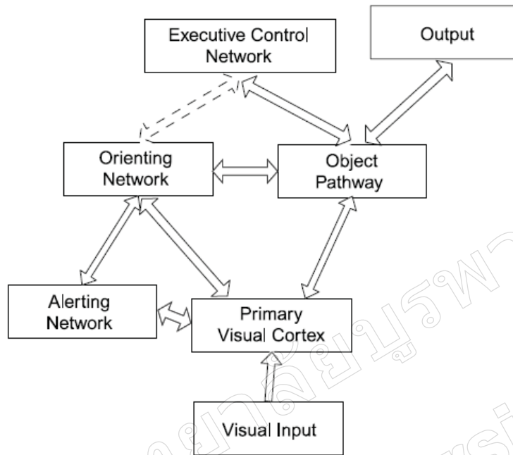
ภาพที่ 3 แผนภาพแสดงความเชื่อมโยงของการเกิดโครงข่ายความสนใจ (Attention network) แต่ละเซลล์ประสาทมีการทำงานเชื่อมกันและตอบสนองต่อหน้าตัวอย่างเดียวกัน (Associated neuronal areas) ทำให้เกิดเป็น neuronal network เมื่อนำมาอธิบายการทดสอบ ANT พบว่าเริ่มต้นจากสิ่งเร้าภาพนอกจากการมองเห็น (Visual input) ส่งผ่านกระแสประสาทไปยังสมองที่เกี่ยวข้องกับการมองเห็น (Primary visual cortex) และทำให้เกิดขั้นแรกของกระบวนการความสนใจ นั่นคือ ความตื่นตัว (Alert) หลังจากนั้นเข้าสู่ขั้นตอนการจัดเรียง (Orient) และส่งไปยังขั้นสูงสุดคือความสนใจในระดับสูง Executive control pathway) ที่ต้องอาศัยมิติการตัดสินใจเรื่องระยะ ทิศทางที่มีเงื่อนไขซับซ้อนมากขึ้น (Spatial-dimension related-conflict) หลังจากการประมวลข้อมูลบูรณาการทางสมองขั้นสูงแล้ว จึงจะทำให้เกิดผลลัพธ์สุดท้ายคือการเกิดการตอบสนองออก (output) (Wang & Fan, 2007)
